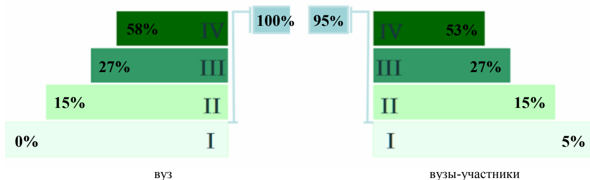
Рисунок 3.47 – Диаграмма распределения результатов тестирования студентов
