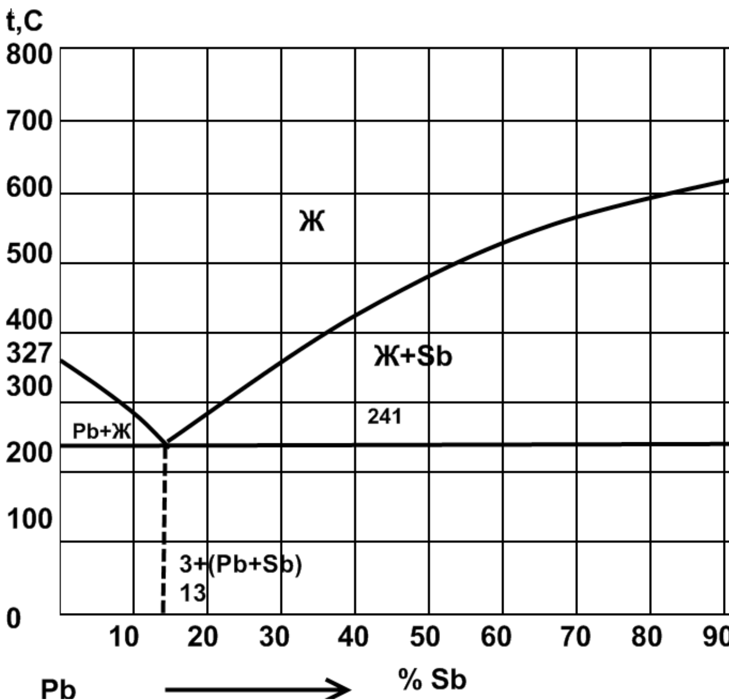
Диаграмма состояния свинец – сурьма (Pb – Sb)
